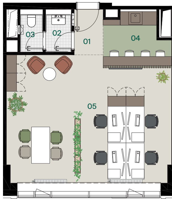
OBRYS BUDOVY
