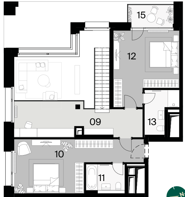
Pôdorys 15p
